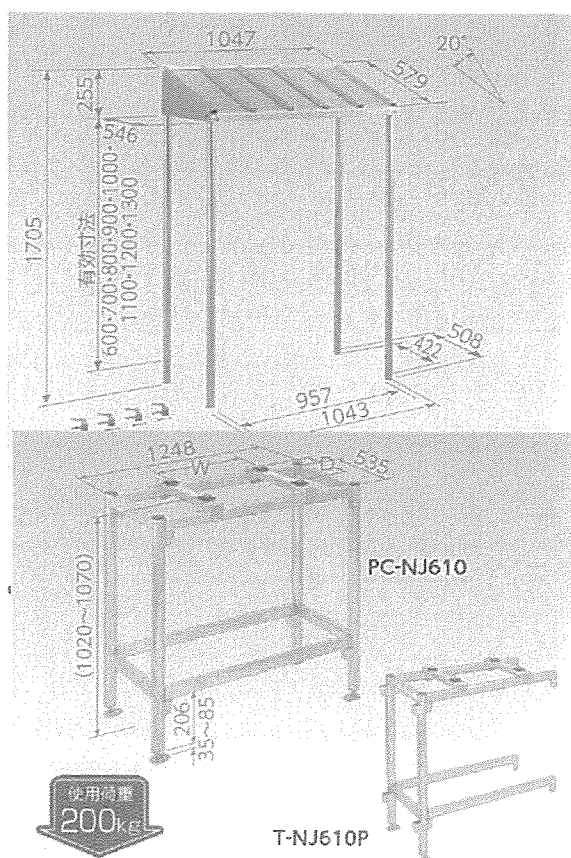
寒冷地向けエアコン屋外機
